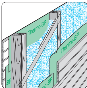
Holzständer mit Nut-Feder-Schale
