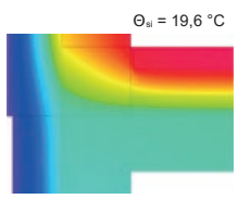
mit Thermo-Fill® Thermo-Floor® verfüllt
