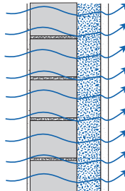
Bild 2b Fassade Kerndämmung
