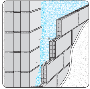
Kerndämmung mit Ziegel-Innenschale verputzt
