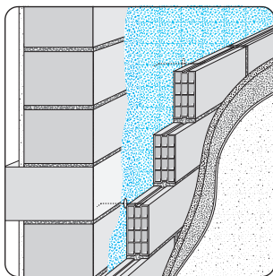
Kerndämmung mit Ziegel-Außenschale verputzt
