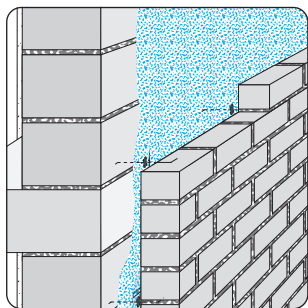
Kerndämmung mit Klinker-Außenschale
